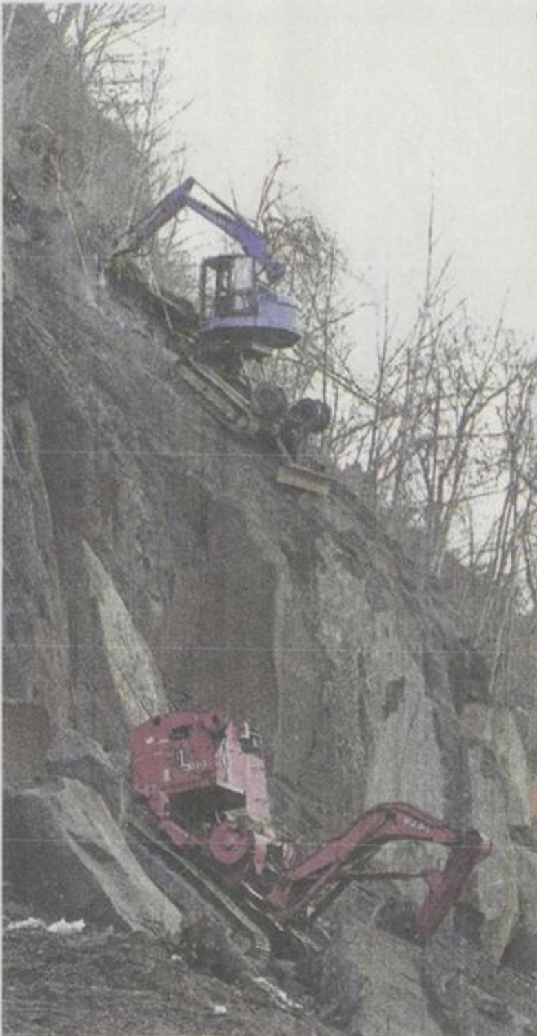
岩盤に張り付いて作業している削岩機。下が無線操縦型
